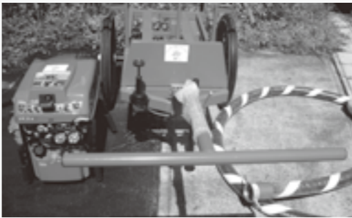
整備された尾続区(登下)の可搬ポンプ
