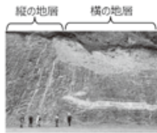
秋山の旧榎井小学校の押されて折れ曲がった地層
